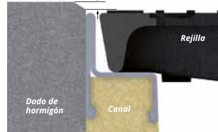
Detalle A Canal con Perfil 3-5mm desde el perfil
