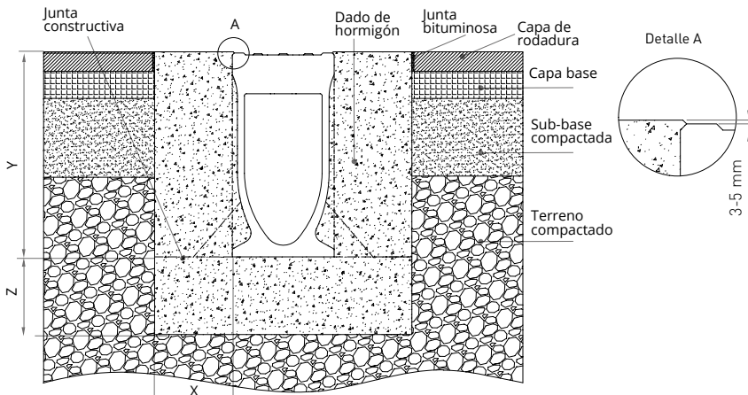
D400 - E600 - F900 Longitudinal a la dirección del tráfico
