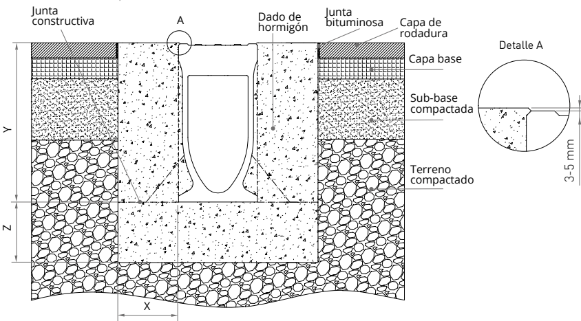
D400 - E600 - F900 Transversal a la dirección del tráfico
