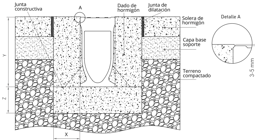
D400 - E600 - F900 Longitudinal a la dirección del tráfico
