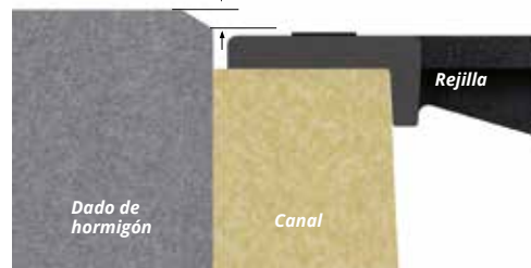
Detalle B Canal sin Perfil 3-5mm desde la rejilla
