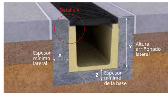
Detalle A Canal con Perfil 3-5mm desde el perfil
